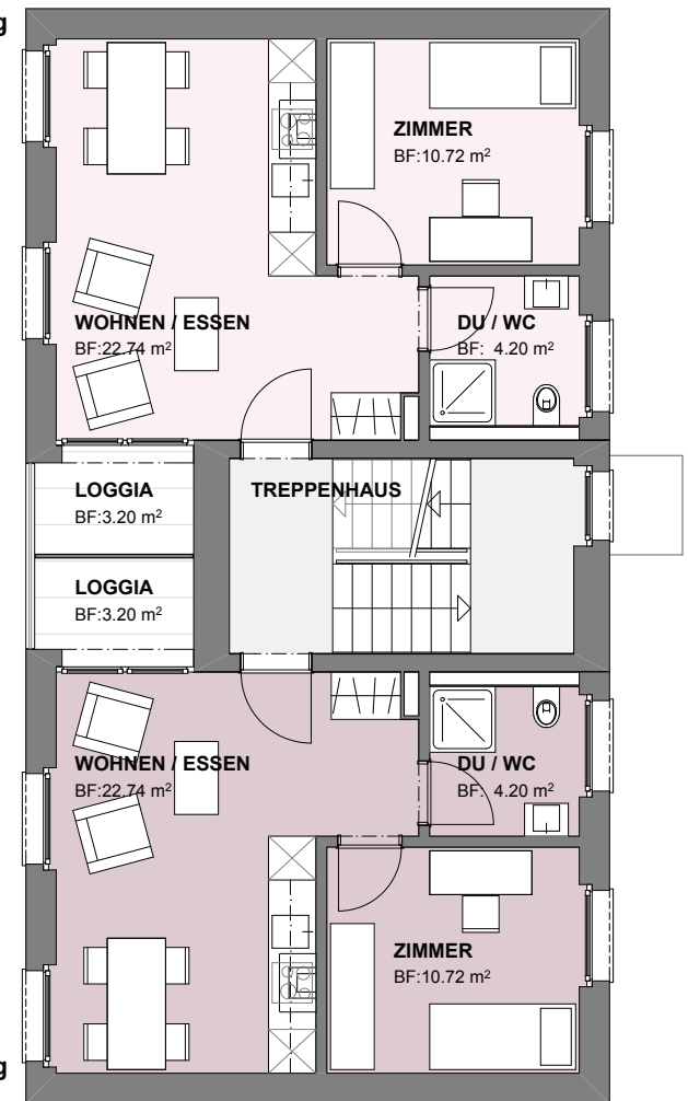
1-½ Zimmer Wohnung C | 3.OG.w07
