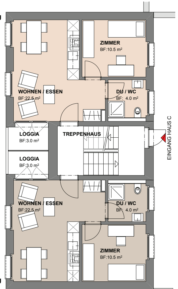
1-1/2 Zimmer Wohnung C | EG.w01
