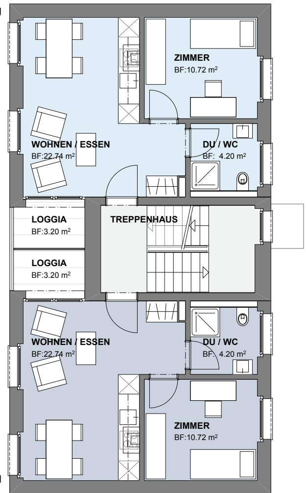
1-½ Zimmer Wohnung C | 2.OG.w05
