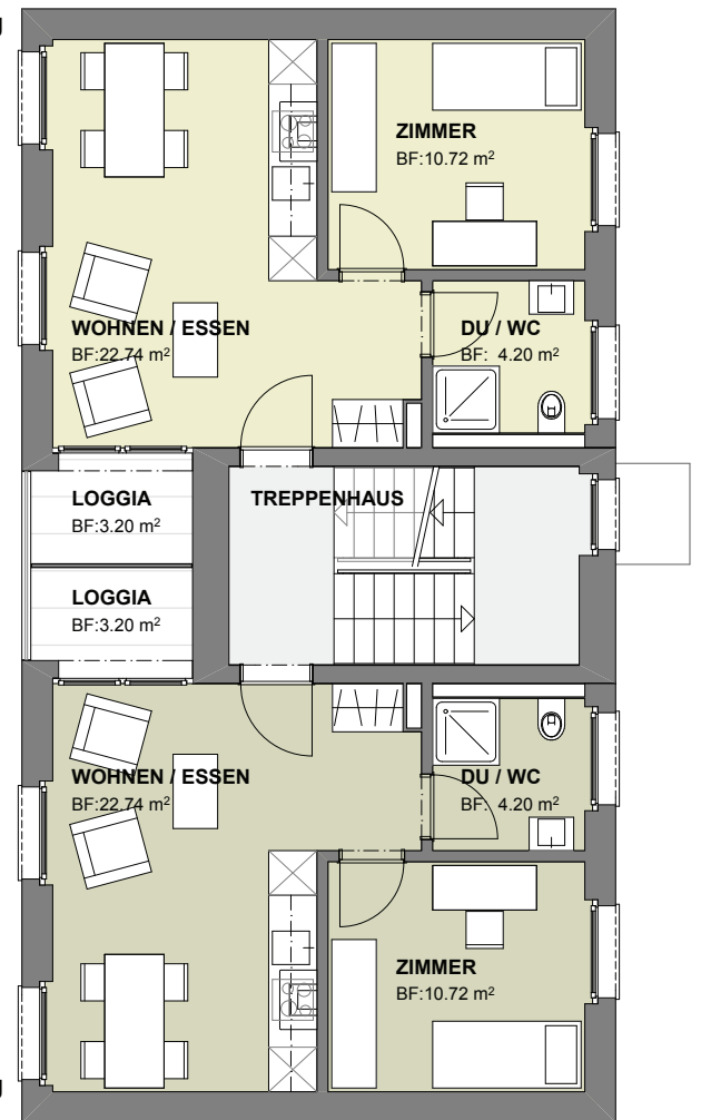
1-½ Zimmer Wohnung C | 1.OG.w03
